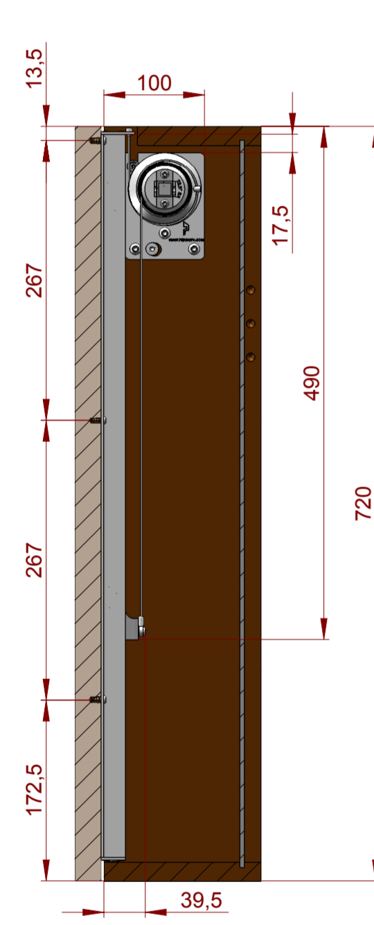
SEZIONE B-B
