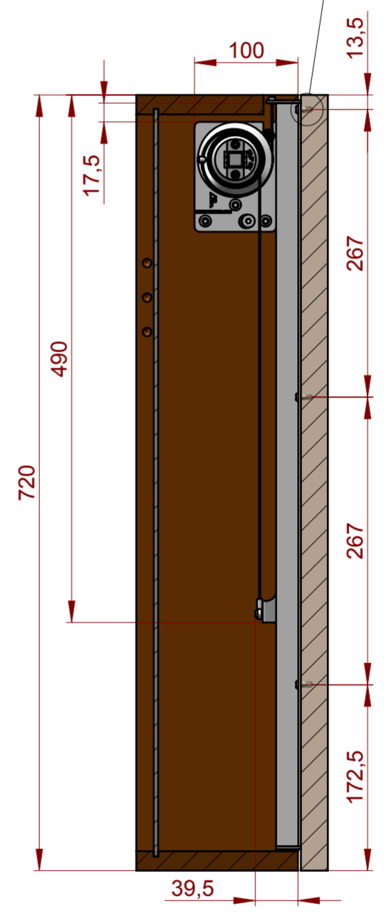
SEZIONE A-A
