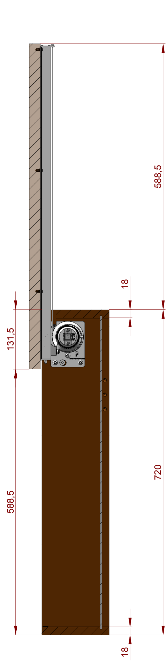
SEZIONE D-D
