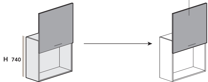
Altezza / Height H. 740 mm
