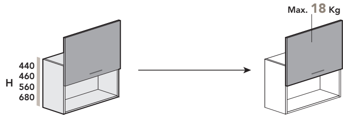
Altezza / Height H. 440 mm - 460 mm H. 560 mm - 680 mm
