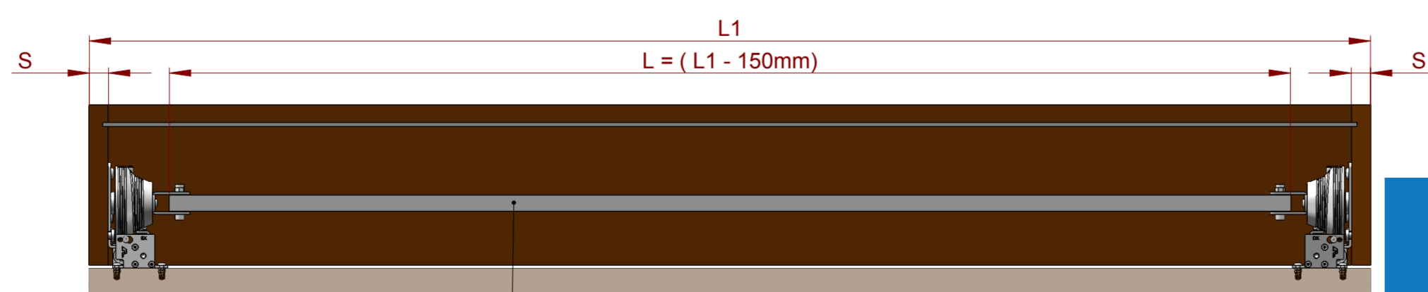
Codice / Code : 619XXX14 (Vedi Tabella / See Table)
