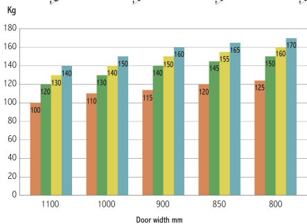
Load capacity chart 負重表
