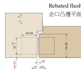
Door cross section 門橫截面
