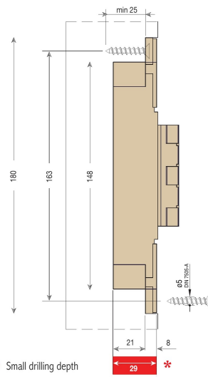
Hinge dimensions 鉸鏈尺寸
