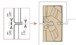
Hinge dimensions 鉸鏈尺寸
