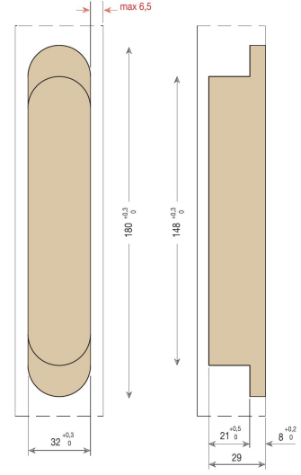
Cutout dimension 開槽尺寸
