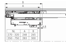
Position of the synchronization rod 同步橫杆位置
