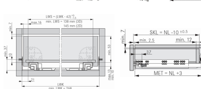
Installation dimension 安裝尺寸
